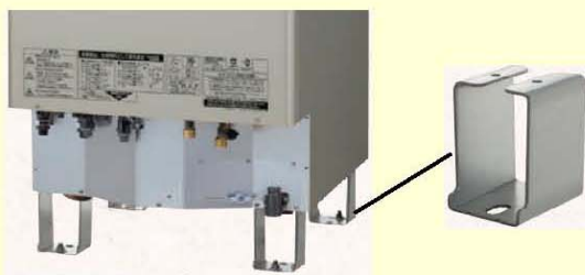
揺れが脚部の一部に集中しにくい 一体構造の足4本で本体をしっかりと支える 耐食性の高いZAM銅板を脚部に採用
